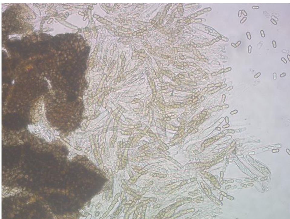
SLIKA 2. ZRELE ASKOSPORE Venturia inaequalis
